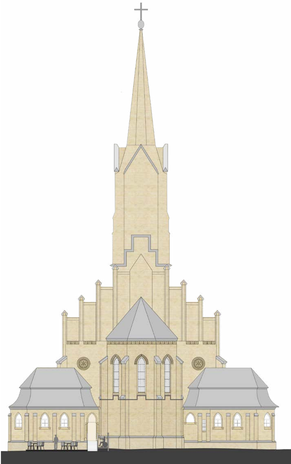
Ansicht Nord/Ost
