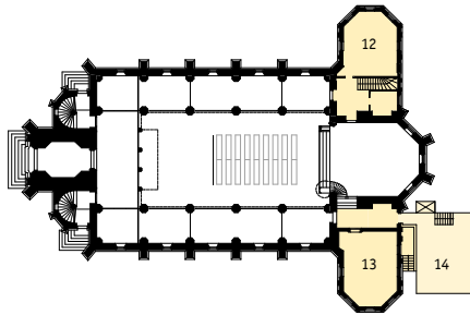
Bauphase 2 EG
