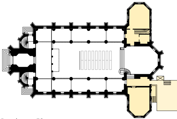
Bauphase 2 EG
