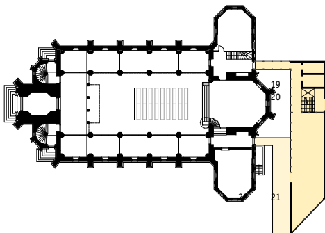
Bauphase 3 EG
