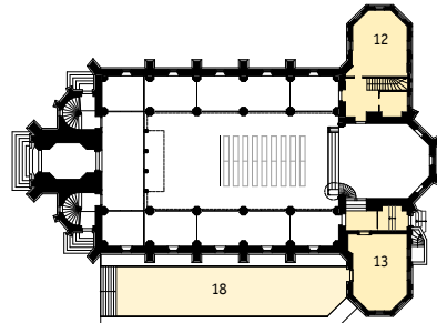
Bauphase 2, Variante 2b EG
