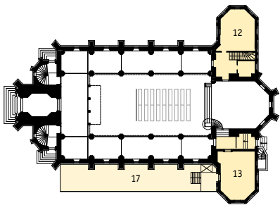
Bauphase 2, Variante 2a EG
